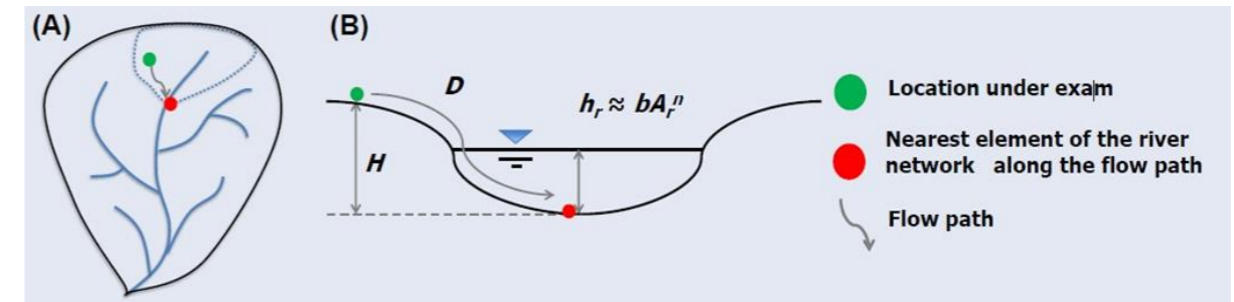
Gambar 3. 4. Potongan Melintang Deskripsi Metodologi GFI
