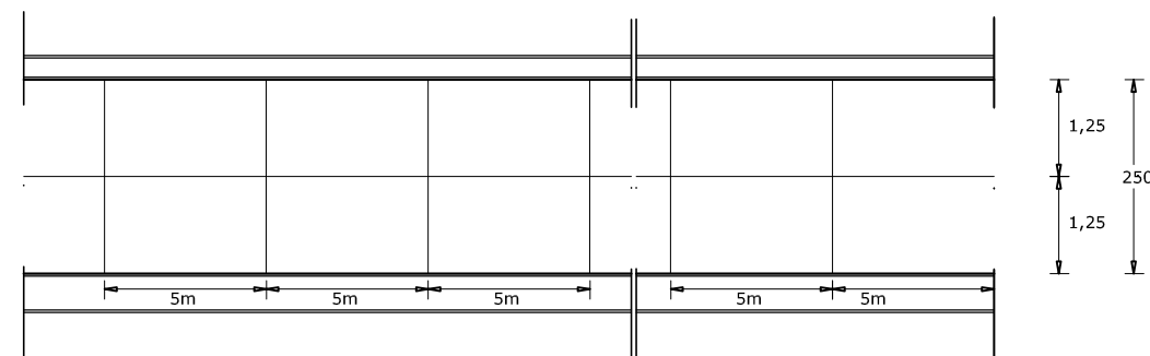
DENAH PEMBAGIAN SEGMENT SKALA 1:500
