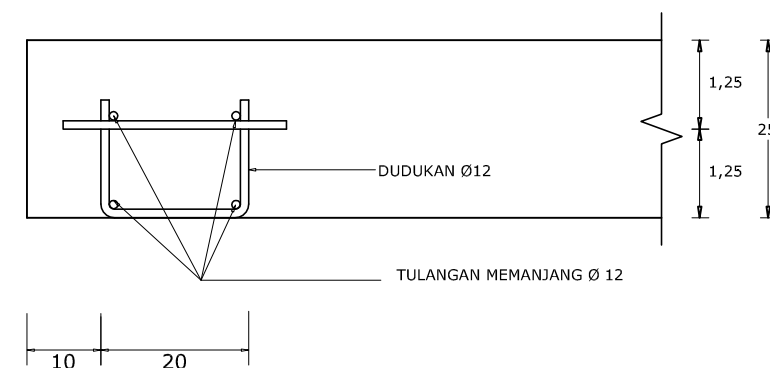
PENULANGAN TEPI SKALA 1:10
