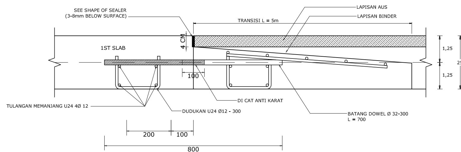
TRANSISI STRUKTUR DENGAN PERKERASAN ASPAL SKALA 1:10
